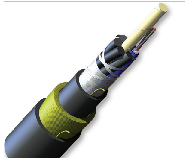
Part Number: 012KAE-T4E30A20
