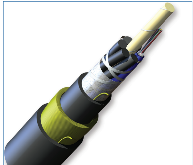
Part Number: 012TAE-T4C31A20
