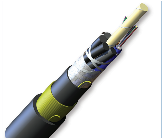
Part Number: 024EAE-T4201A20
