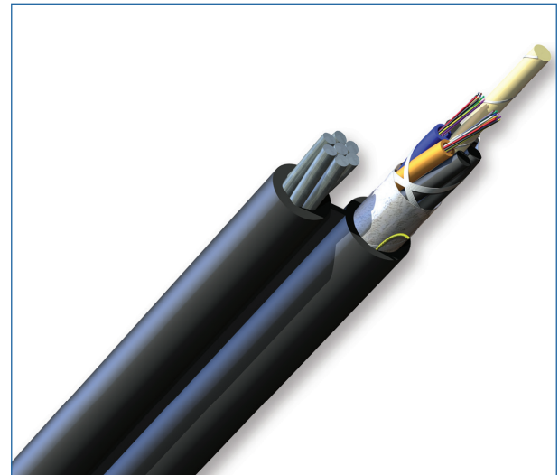
Part Number: 024EUA-T4101D20
