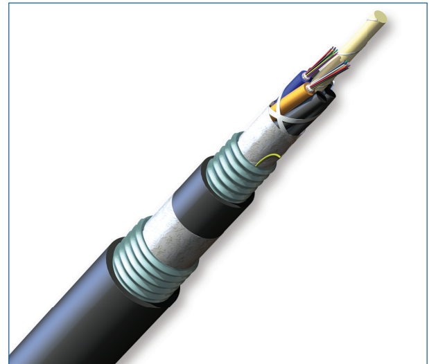
Part Number: 024TUD-T4131A20
