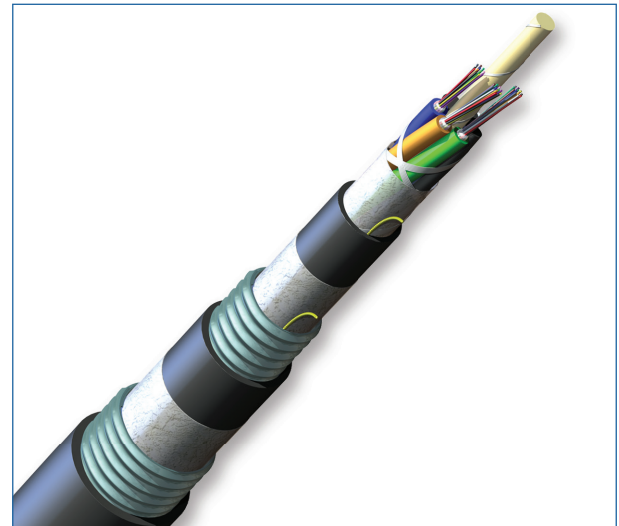
Part Number: 036KU6-T4130A20
