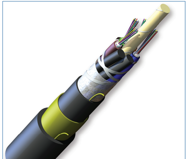
Part Number: 048KAE-T4230A20
