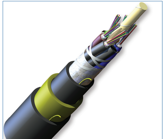
Part Number: 060EAE-T4C01A20
