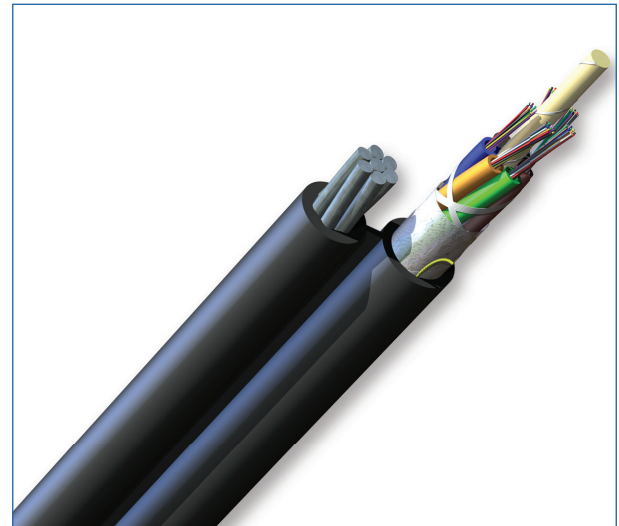
Part Number: 060KUA-T4130D20
