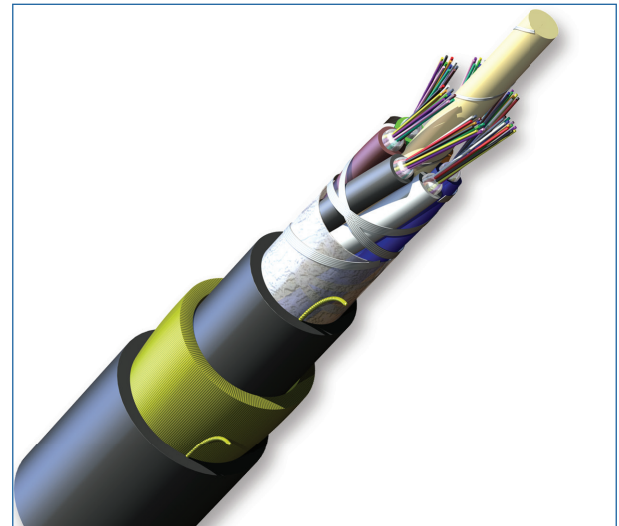
Part Number: 072EAE-T4C01A20
