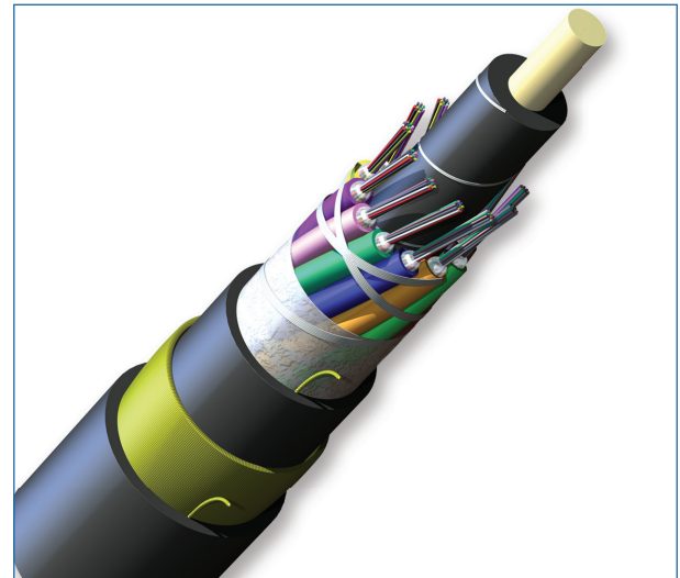
Part Number: 144EAE-T4A01A20
