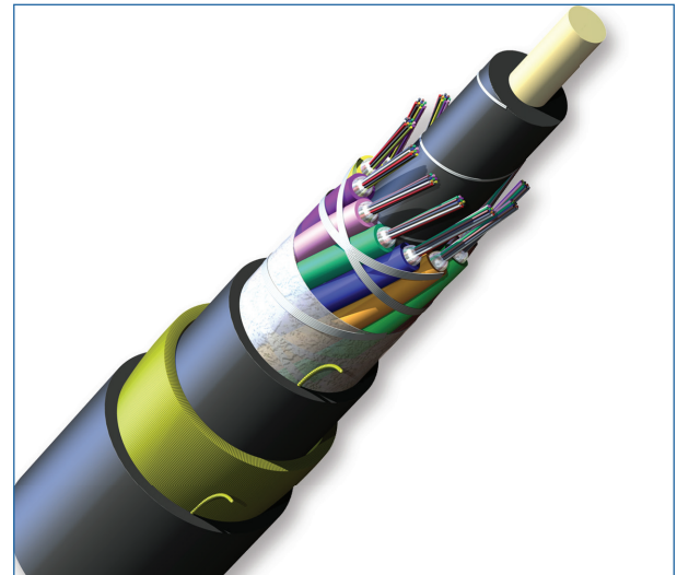
Part Number: 144EAE-T4F01A20
