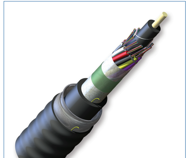
Part Number: 144EUZ-T4101DAN
