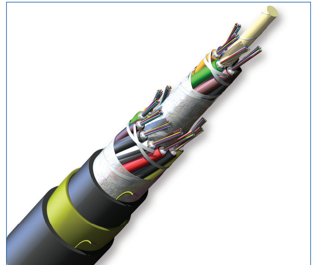
Part Number: 192EAE-T4801A20
