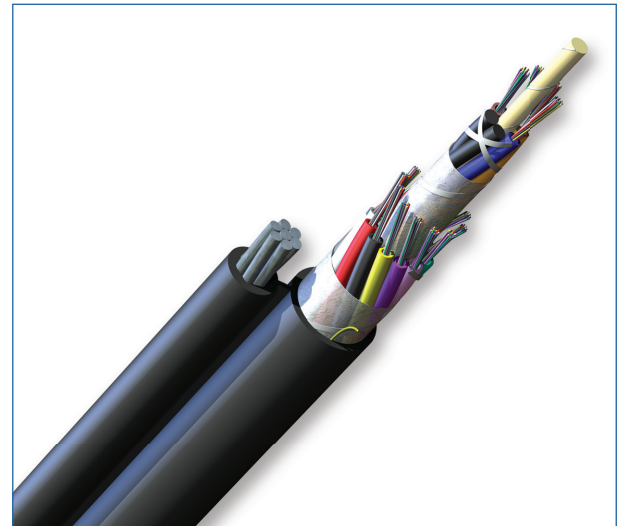
Part Number: 192KUA-T4130D20
