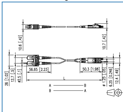
Produktbild 151J1EOJ0XXE (OM3 - SC-D Dimensional drawing
