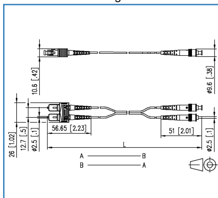
Produktbild 151P1EOAOXXE (OS2 - SC-D Dimensional drawing
