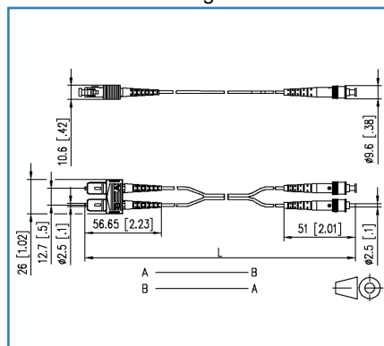
Produktbild 151S1EOAOXXE (OM4 - SC-D Dimensional drawing
