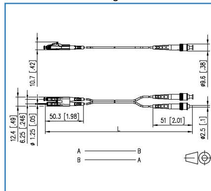
Produktbild 151S1JOAOXXE (OM4 - LC-D Dimensional drawing
